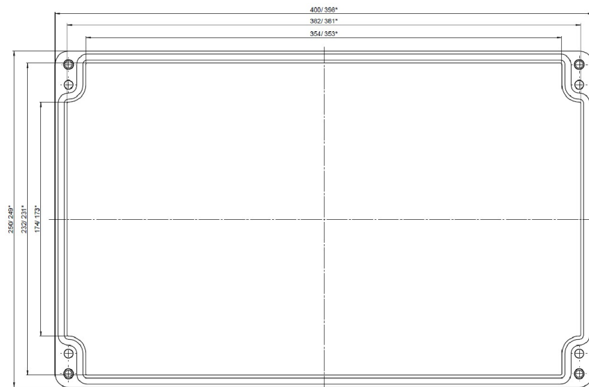
Deckel / Lid
